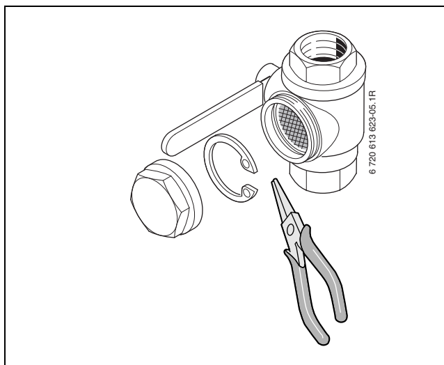
Bild 31 Filtervariant med låsring
