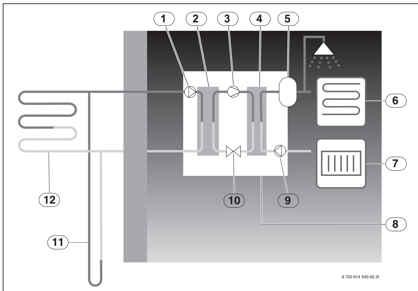
Bild 2 Funktionsbeskrivning
