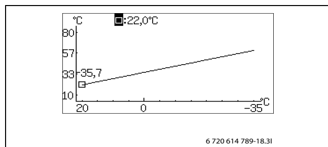
Bild 23 Inställningsfönster Värmekurva (radiator)
