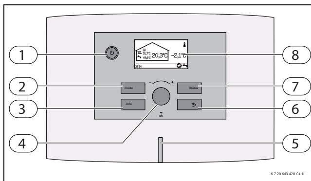
Bild 3 Kontrollpanelen
