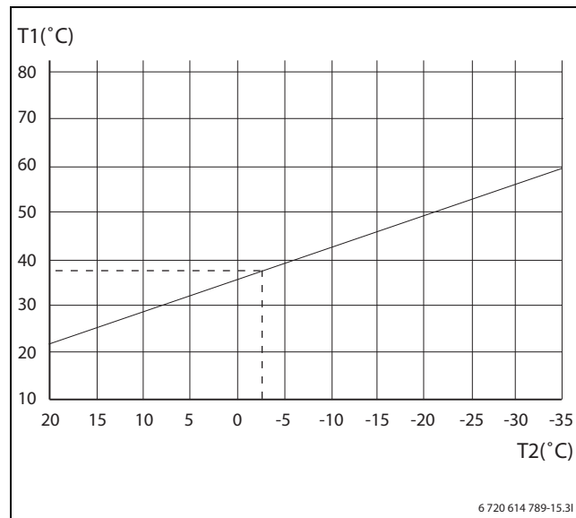
Bild 21 Radiator
